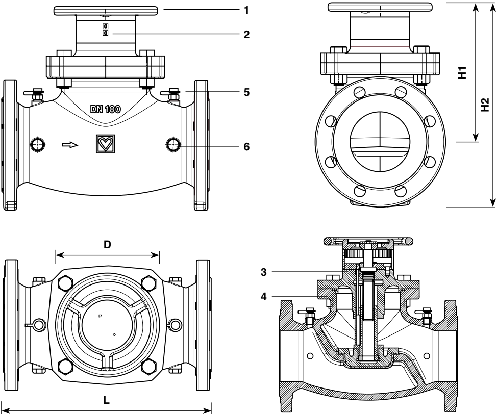
Flanschabmessung nach EN 1092-2
